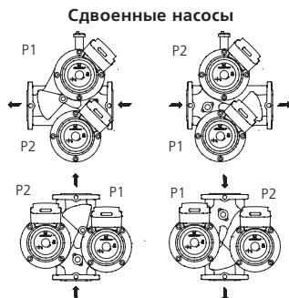
Двоянные насосы
